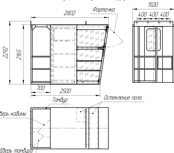
Габаритный чертеж стандартной кабины
